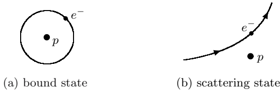
Fig. 2.11. Hydrogen atom
